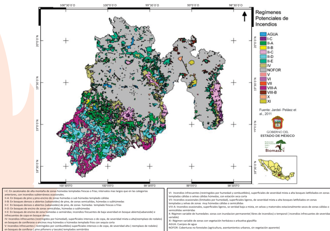
Figura 8. Regímenes potenciales de incendios en el Estado de México
