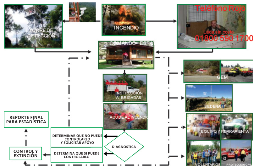
Figura 10. Esquema operativo para el combate de incendios forestales en el Estado de México
