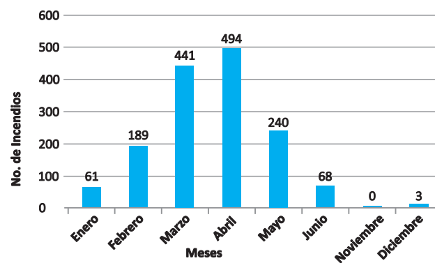
Figura 2. Ocurrencia de incendios forestales por mes del año 2004-2014
