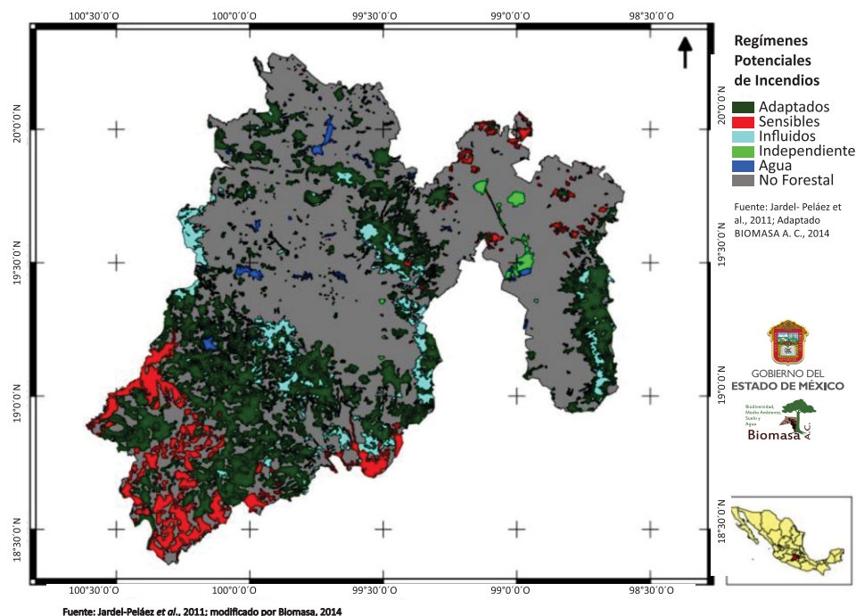
Figura 9. Clasificación de ecosistemas por regímenes potenciales de incendios en el Estado de México
