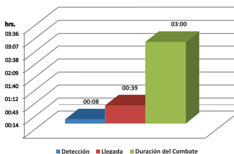
Figura 6. Tendencia de los indicadores de eficiencia en la atención de los incendios forestales, 2004-2014
