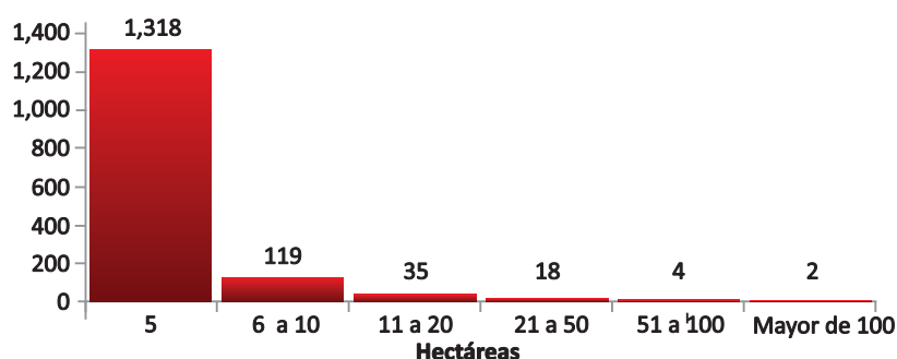
Figura 4. Tamaño de los incendios forestales, 2004-2014
