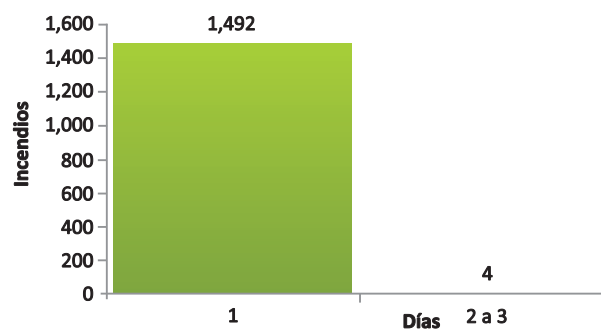
Figura 3. Duración de incendios forestales 2004-2014
