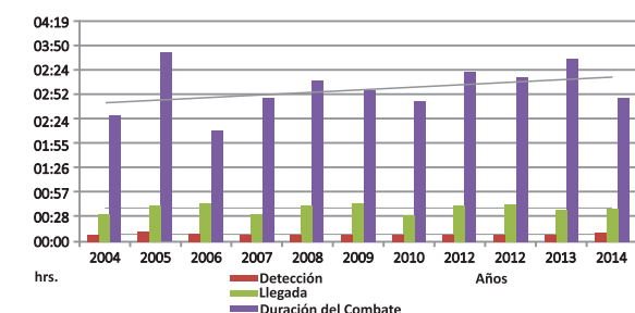
Figura 6. Tendencia de los indicadores de eficiencia en la atención de los incendios forestales, 2004-2014
