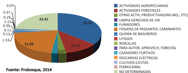
Figura 7. Porcentaje de causas, promedio anual 2004-2014
