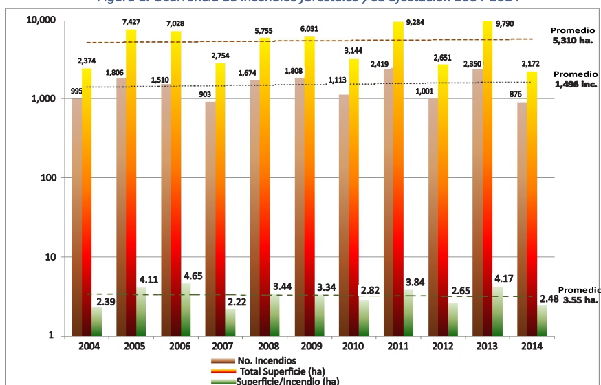
Figura 1. Ocurrencia de incendios forestales y su afectación 2004-2014
